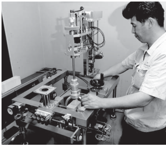
▲機械組立風景
