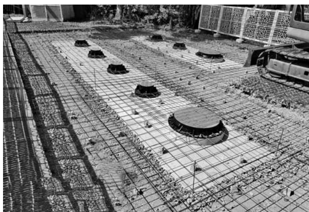
工事中の貯留式トイレ
