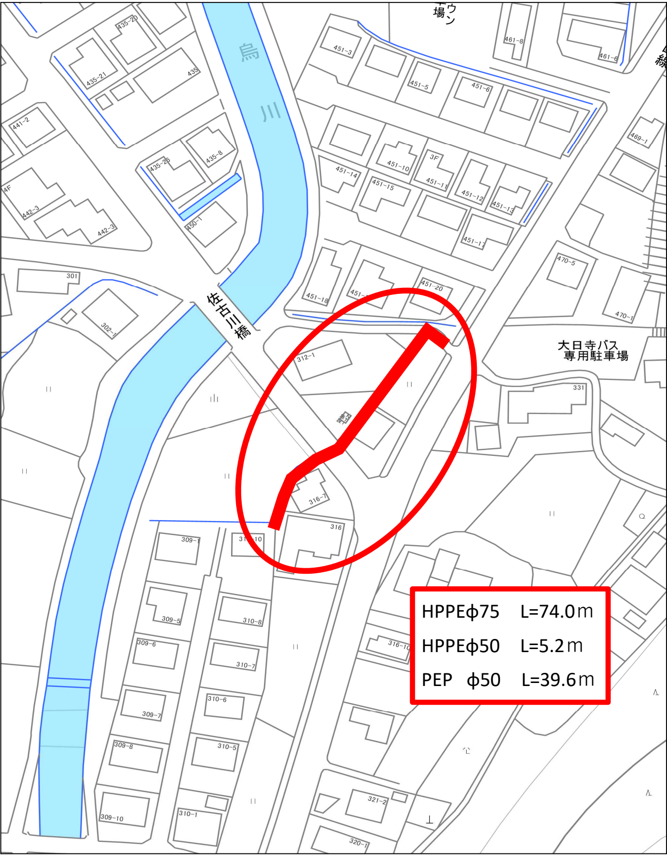
(詳細図)
