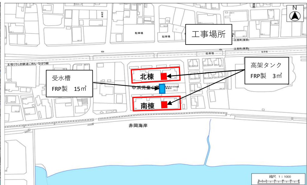
詳細図
