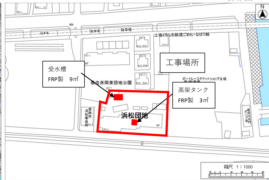
詳細図
