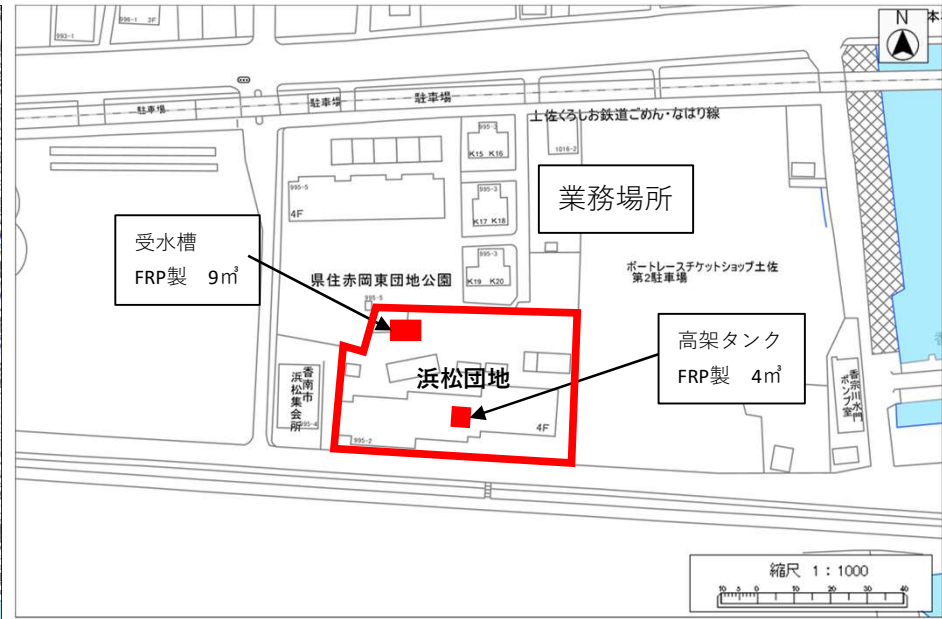
詳細図
