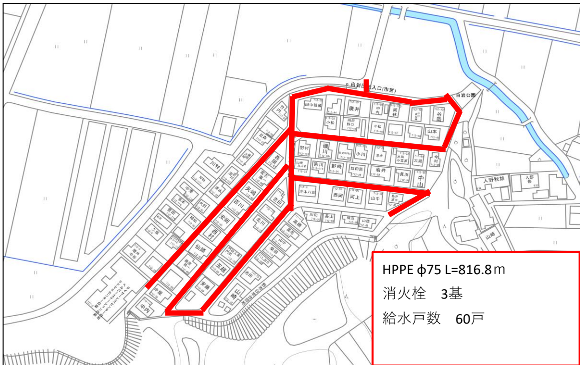
(詳細図)
