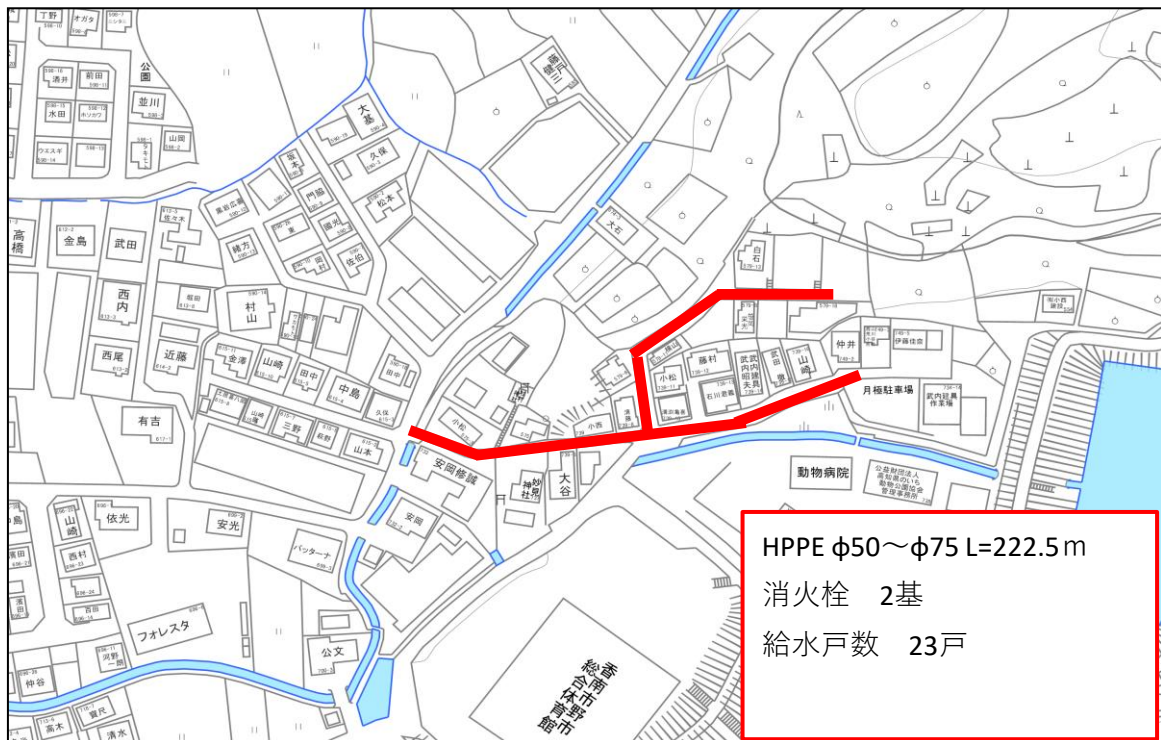
(詳細図)
