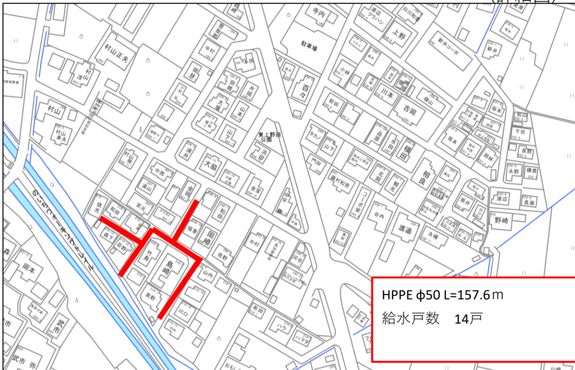
(詳細図)
