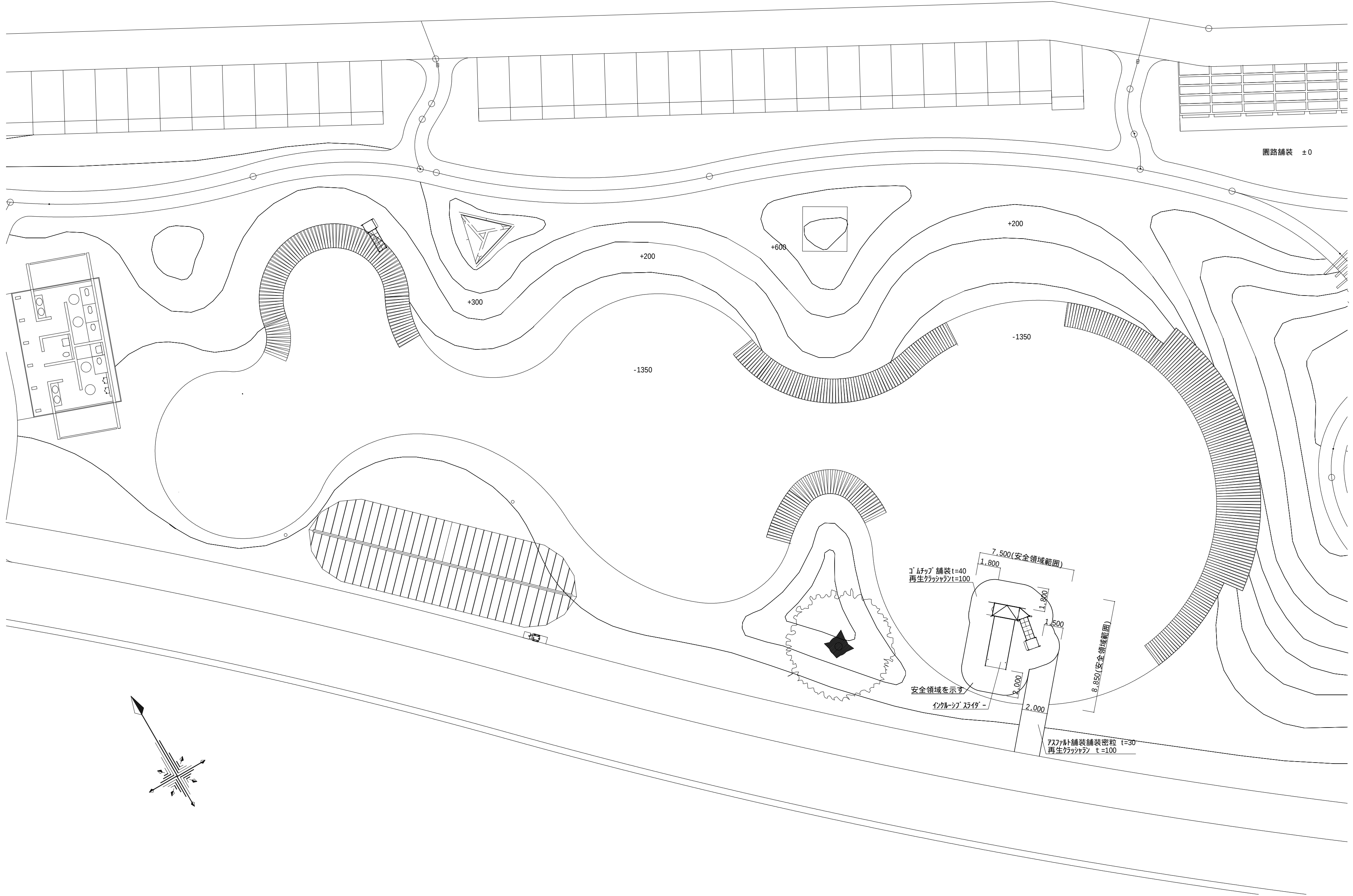
配置図 S=1/200
