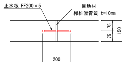
A断面図
