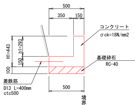
1 号 L 型水路 材量表
