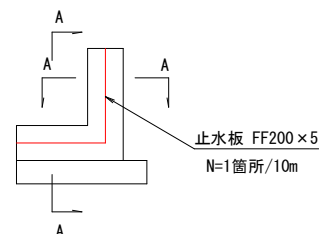
A断面図
