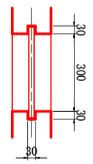
角落し詳細図 S=1:10
