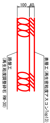
舗装工 S=1:10
