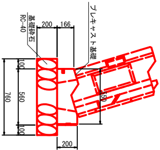
基礎工 S=1:20
