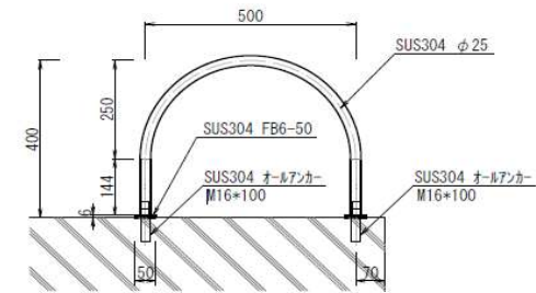
側面図
