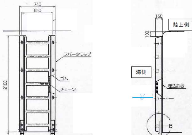
ゴム製タラップ詳細図
