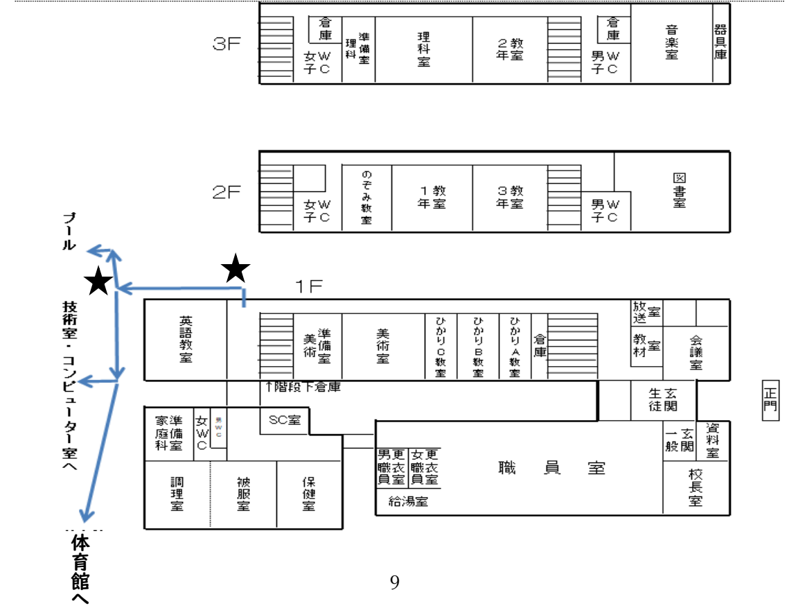
別図第 1（校舎内避難経路） ★誘導員
